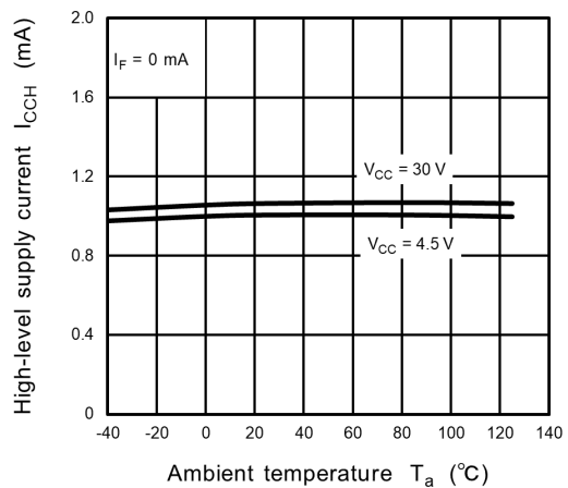
Fig. 12.2.6 I_{CCH} - T_a
