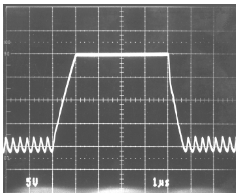
C) AD712
