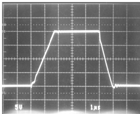
B) LT1057
