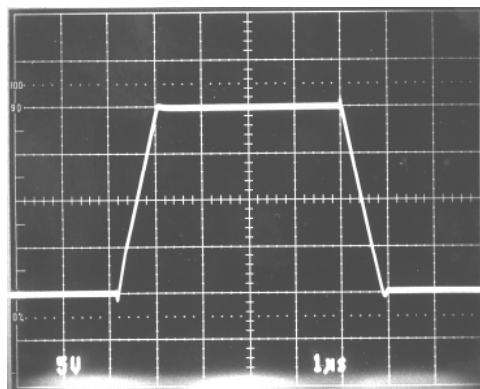
A) OP249
