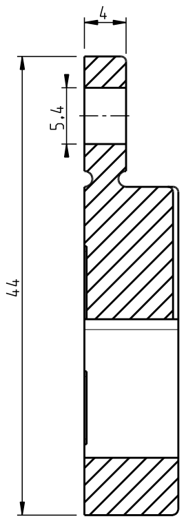
SECT A-A
