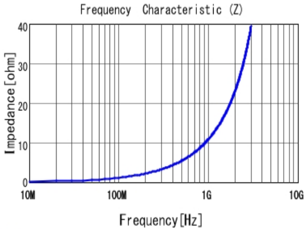
■ LQG15HS1N8S02 |Z|
