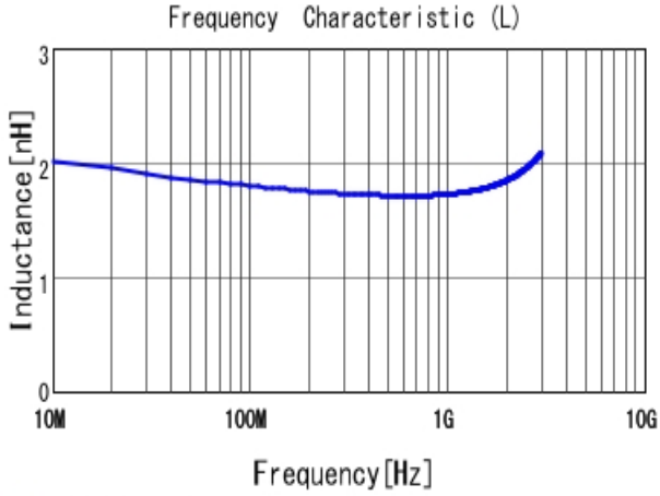
■ LQG15HS1N8S02 L
