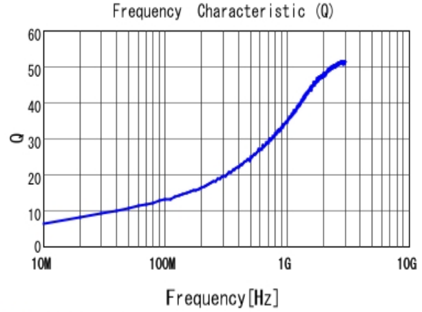
■ LQG15HS1N8S02 Q
