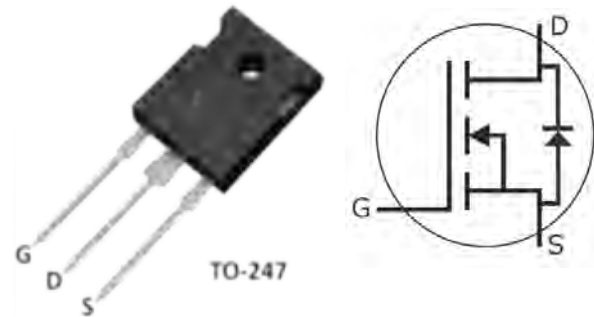
TO-247-3L
