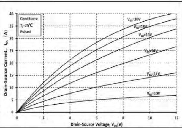
图.2 输出曲线 @ T_j = 25^\circ\text{C}
