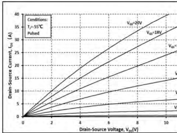
图.1 输出曲线 @ T_j = -55^\circ\text{C}
