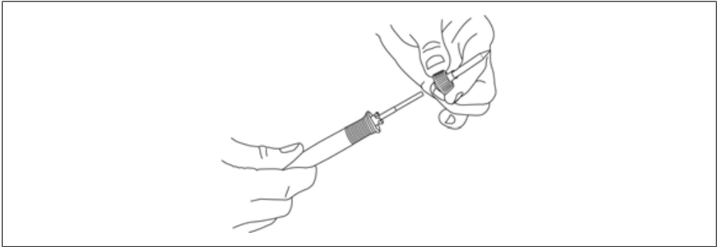
図2: はんだごて先を取り外します
