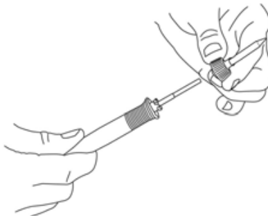
Afb. 1: Ontgrendel de soldeerstift [1] en trek hem eraf [2]
