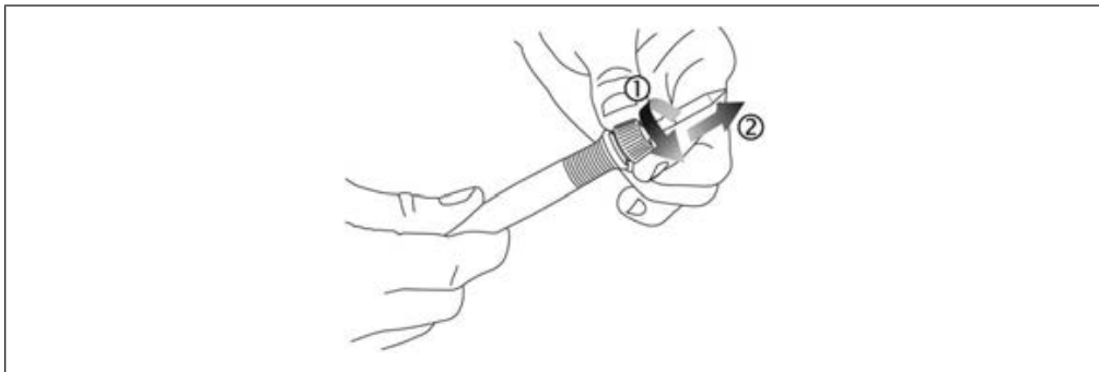
Fig. 1: Débloquer la panne à souder [1] et l'extraire [2]
