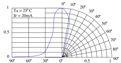
Directivity(Angle:25°) 发光角度 25°
