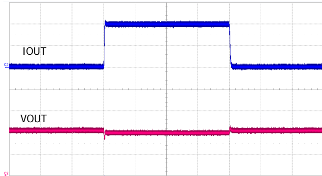
IOUT : 1.0A/div, VOUT : 100mV/div, Time : 500μs/div
